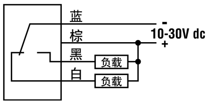
电缆式NPN输出
