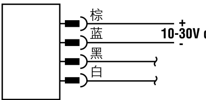
接插件式直流发射器
