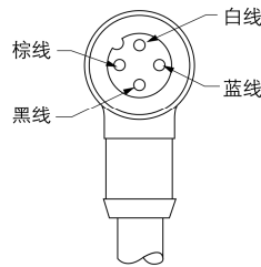
4芯Euro型接插件出线图 (电缆端)
