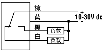
电缆式PNP输出
