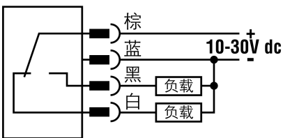
接插件式PNP输出
