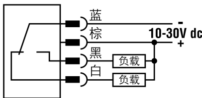
接插件式NPN输出
