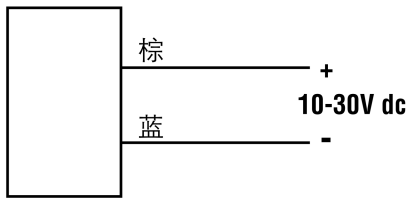
电缆式直流发射器
