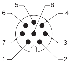
电缆/外壳上的M12插头视图
