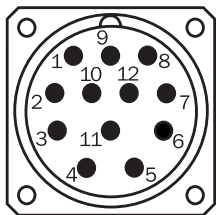
电缆/外壳上的M23插头视图
