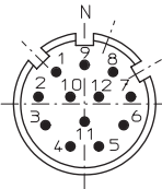
12 针式连接座俯视图:
