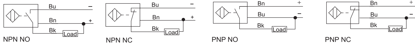
电缆接线
