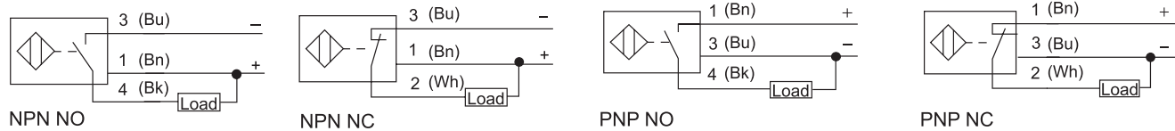
接插件接线
