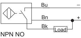
电缆接线
