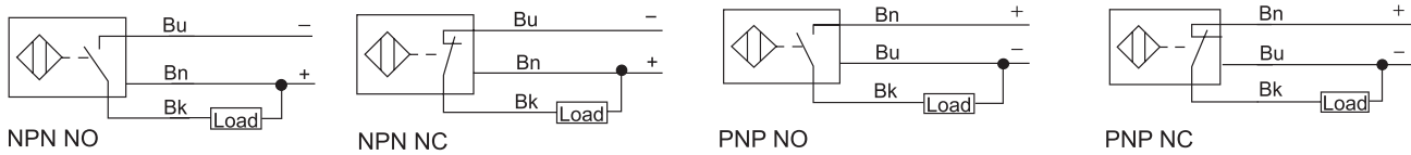
电缆接线
