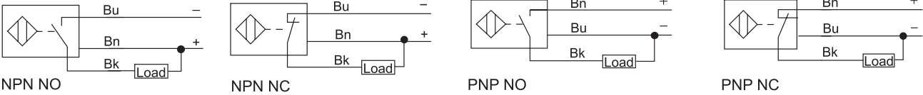
电缆接线
