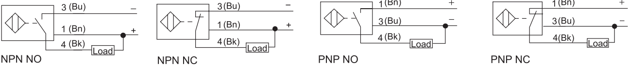
接插件接线
