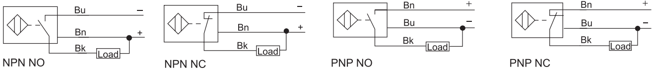
电缆接线
