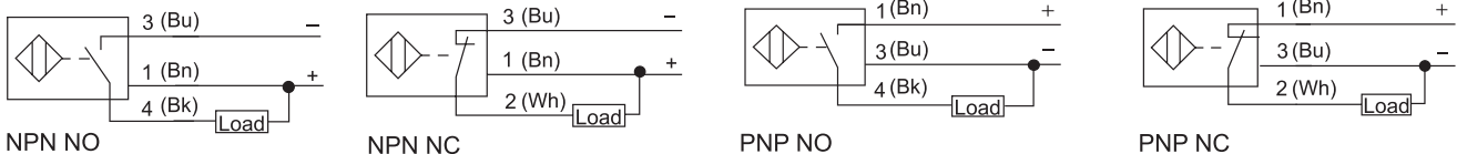
接插件接线
