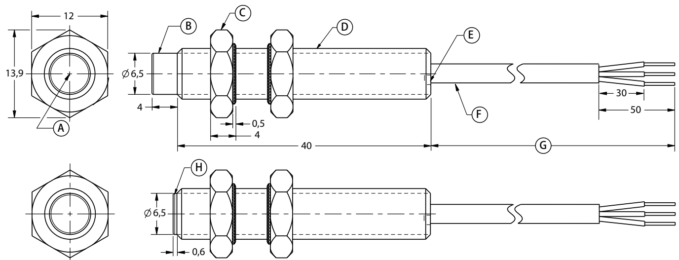
图 9: JSM8 系列安装尺寸 ( 仅供参考: mm )
