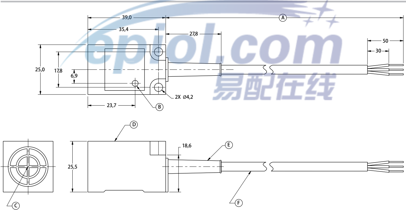
图 6：JPA25 系列安装尺寸（仅供参考：mm）
