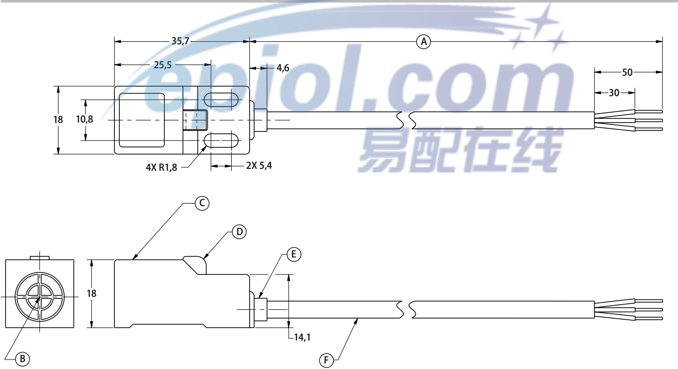
图 5: JPA17 系列安装尺寸 ( 仅供参考: mm )
