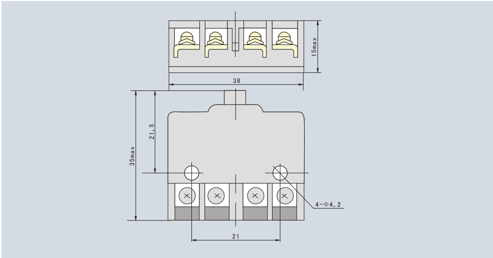
1、LX19K尺寸图
