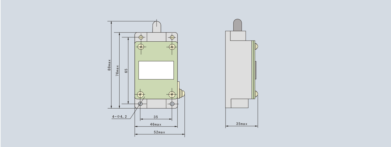
2、LX19-001尺寸图
