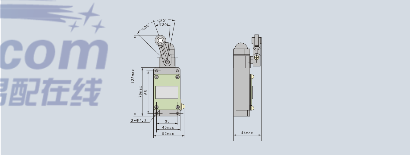
3、LX19-111、121M尺寸图
