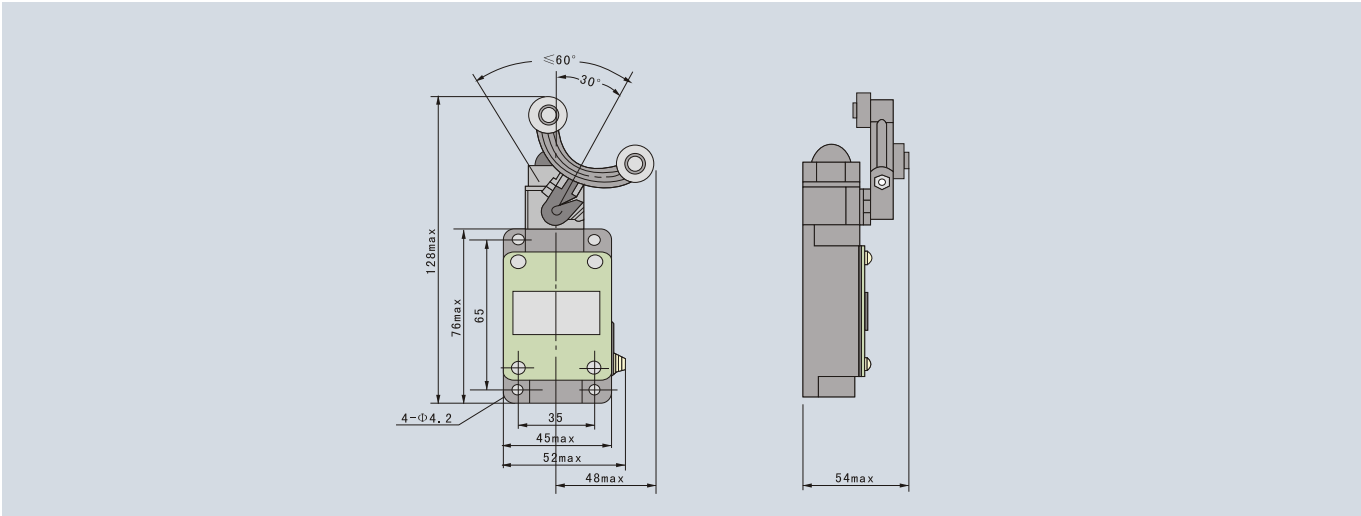
4、LX19-212、222、232尺寸图
