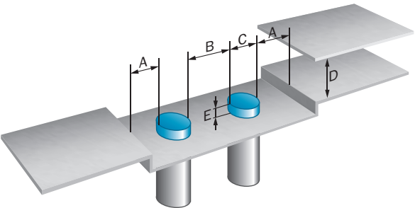
非齐平安装
