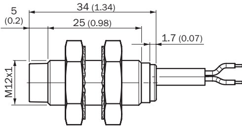
IMB12短外壳, 电缆连接, 非齐平安装
