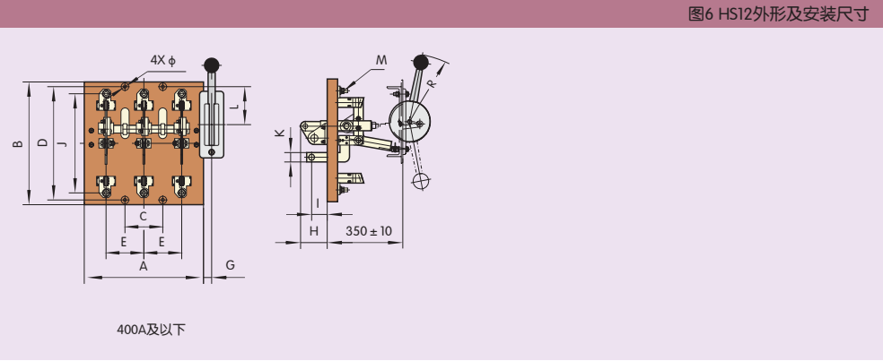
5.6 HS12外形及安装尺寸(见图6、表7)。
