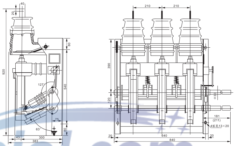
注：用户特殊要求主轴端带 \Phi 10 孔则尺寸为870mm 图1 FN12-12型户内高压交流负荷开关外形图
