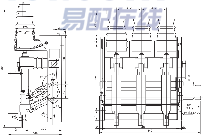
注：用户特殊要求主轴端带 \Phi 10 孔则尺寸为870mm 图2 FNR12-12负荷开关---熔断器组合电器的结构示意图和外形、安装尺寸图
