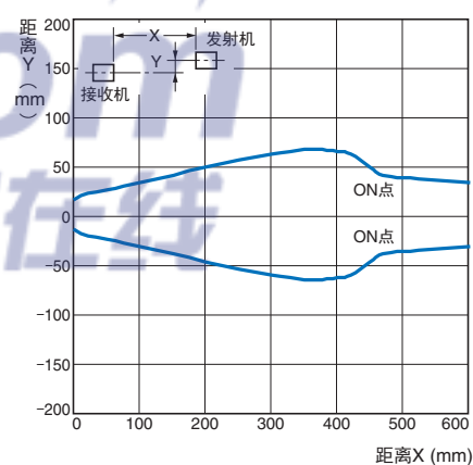
平行移动特性
