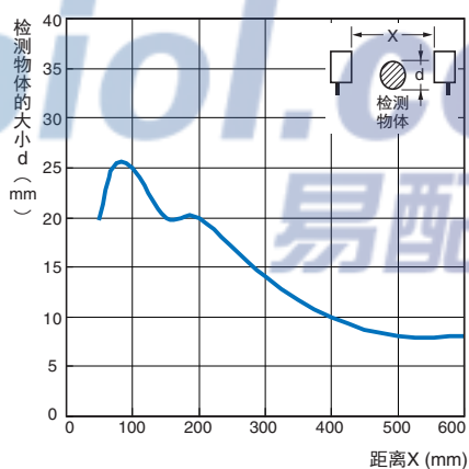
检测距离与检测物体的大小
