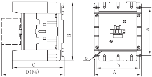
图3 CJX2-115~170外形及安装尺寸
