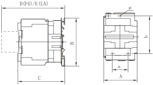
图2 CJX2-40-95外形及安装尺寸
