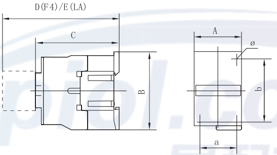
图1 CJX2-09-32外形及安装尺寸
