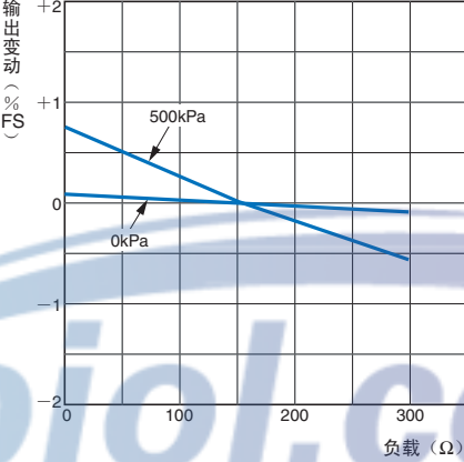
输出电流变动—负载特性 E8AA-M05
