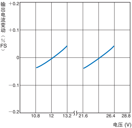
输出电流变动—电压特性 E8AA-M10
