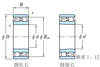
NN 型
