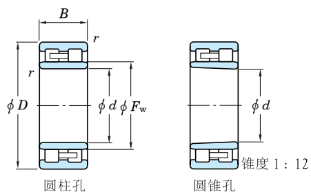
NNU 型
