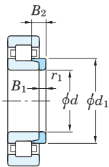
L形挡圈
