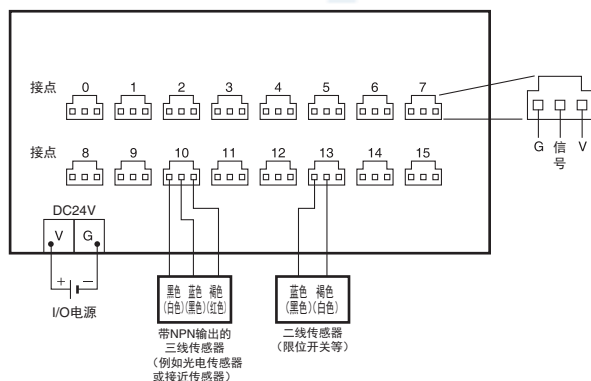
GT1-OD16MX
