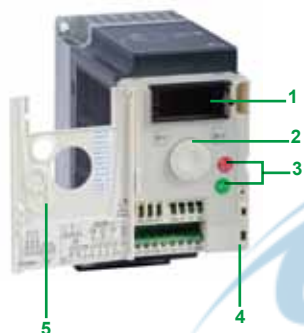
ATV303H037N4 带有门盖的前面板
