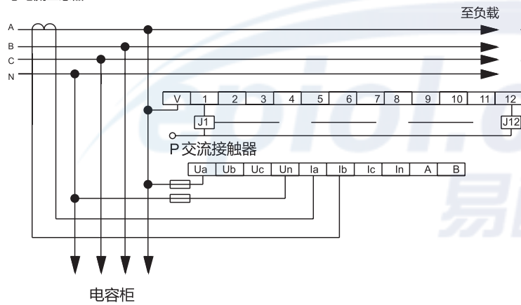
图4 JKG2B(JKW5B)接线图(取样电压220V) 开孔尺寸: 162X102 ( mm )
