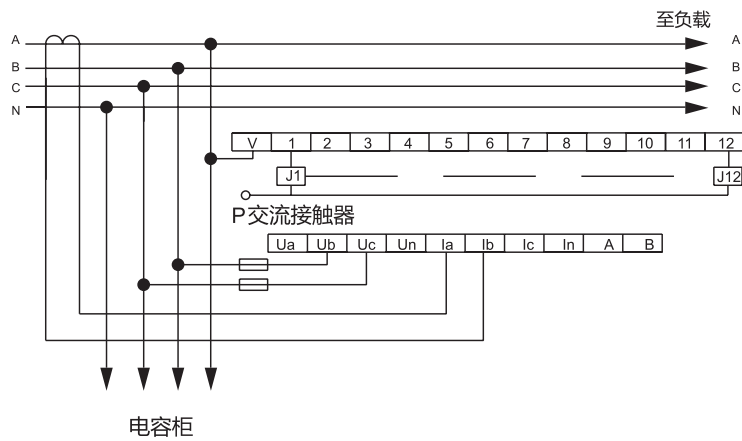
图3 JKG2B(JKW5B)接线图(取样电压380V)
