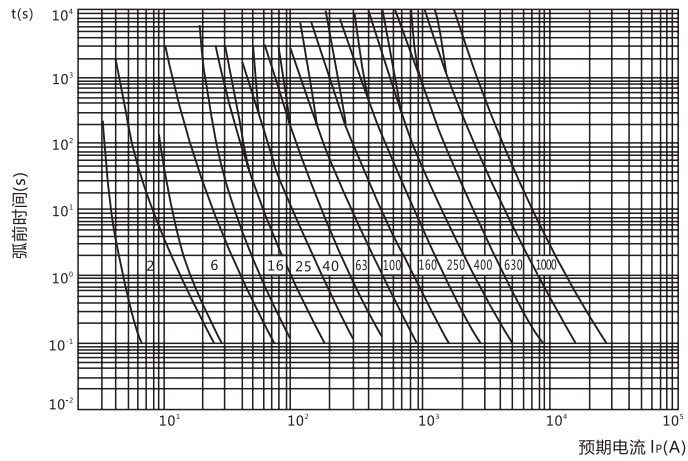
熔断体时间-电流特性曲线
