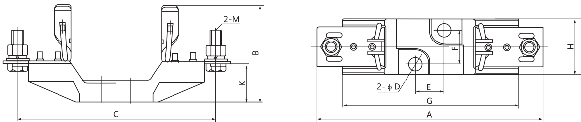
7.2 底座外形及安装尺寸
