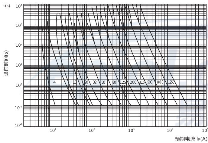
熔断器截断电流特性曲线
