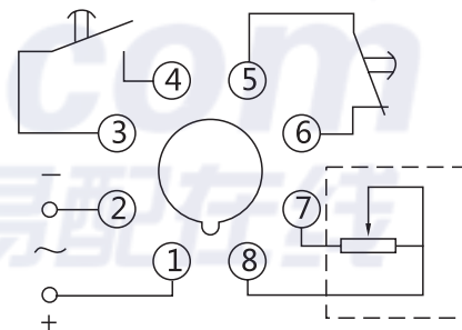
图2 JS14Y接线图
