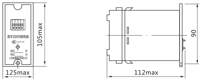
图3 JS14A/M 外形尺寸
