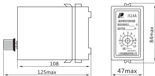
图1 JS14A外形尺寸
