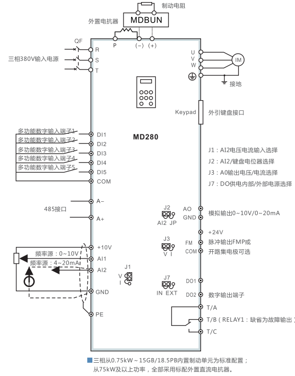
MD280典型接线示意图
