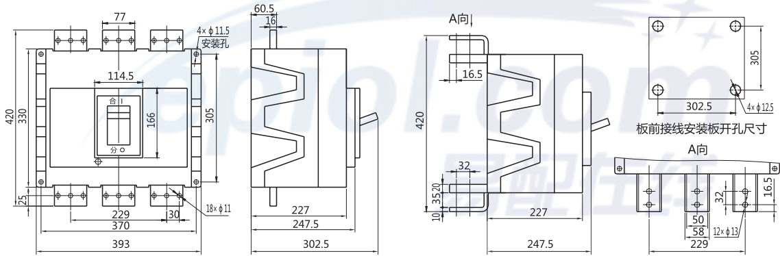
板前接线外形尺寸和安装尺寸
