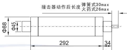
■XRNT1-12/200 熔断体的外形尺寸 单位: mm
