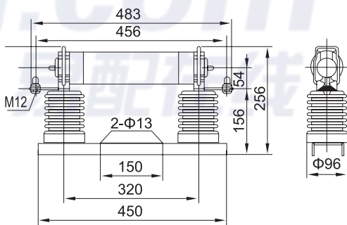
■XRNT1-12 熔断器底座的外形尺寸 单位: mm
