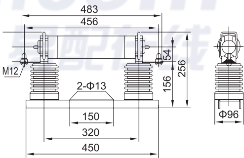
■XRNT1-12熔断器底座的外形尺寸
