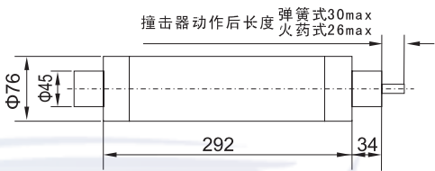
■XRNT1-12/125熔断体的外形尺寸
