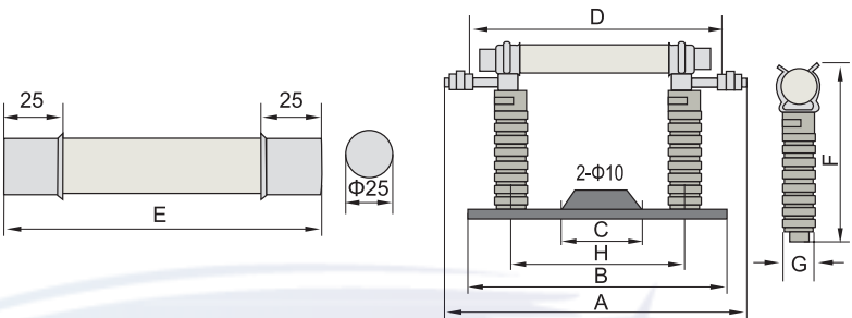
熔断器的外形及安装尺寸
