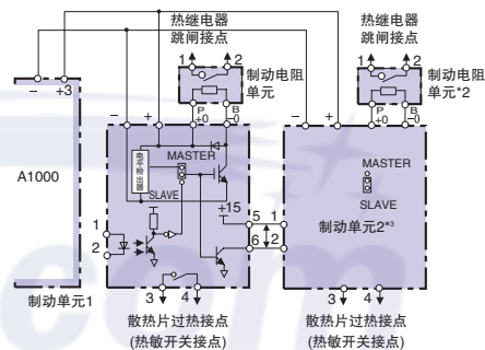
接线图D
