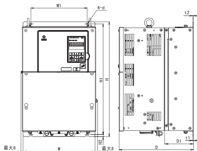
外形图1
