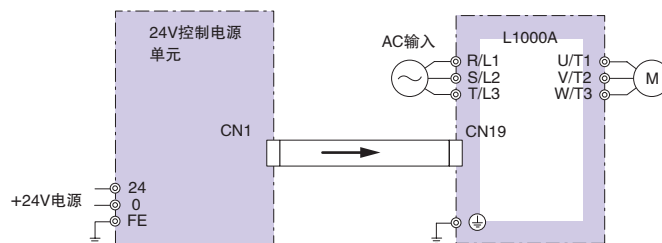
接线图
