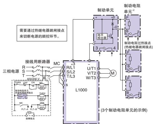
接线图E
