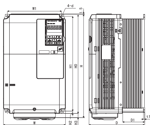
外形图2
