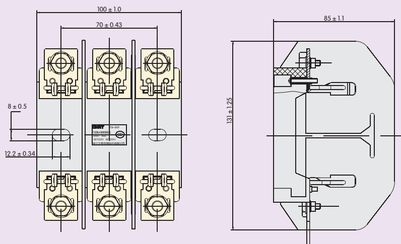
RT36-00-3P外形及安装尺寸图
