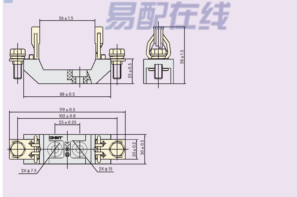
图2 RT36N-00支持件外形尺寸
