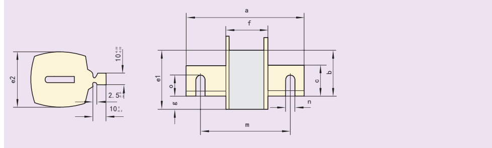
图1 熔断体外形尺寸
