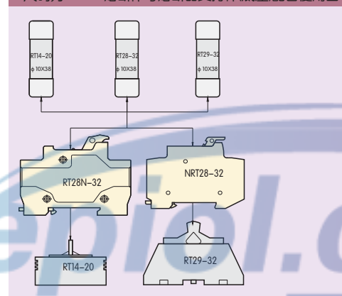
尺码为10×38熔断体与熔断器支持件(底座)配合使用图
