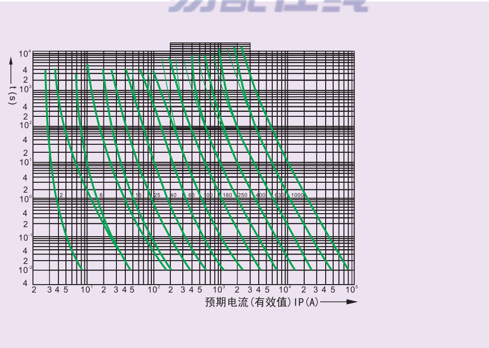
(N)RT36系列刀型触头熔断器特性曲线
