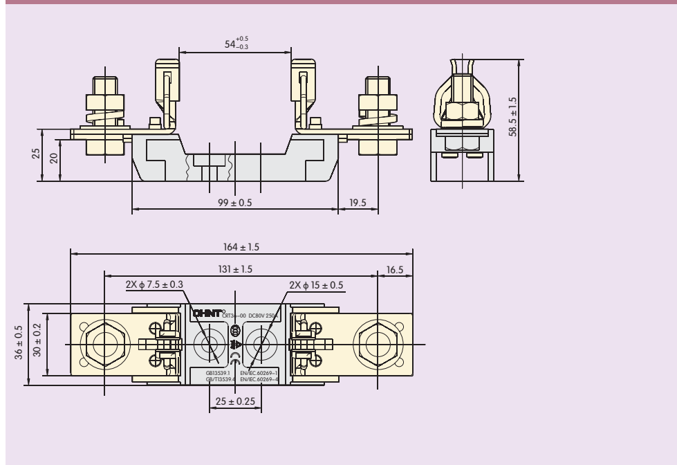
图3 CRT36-00 600(400)A250A底座外型及安装尺寸
