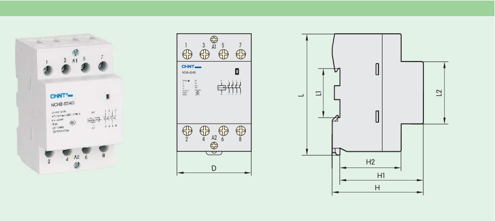
接触器的外形及安装尺寸见表5
