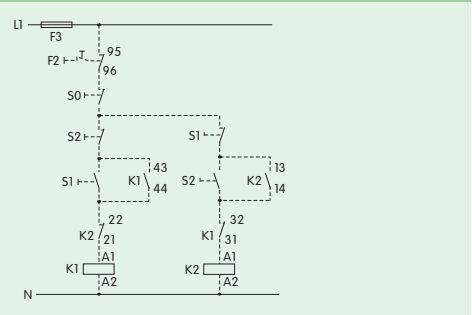
图2 瞬动接触控制的控制回路
