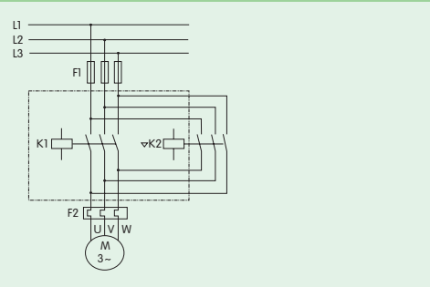
图1 主回路
