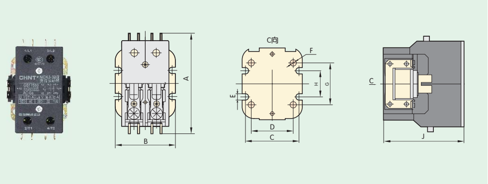
外形及安装尺寸
