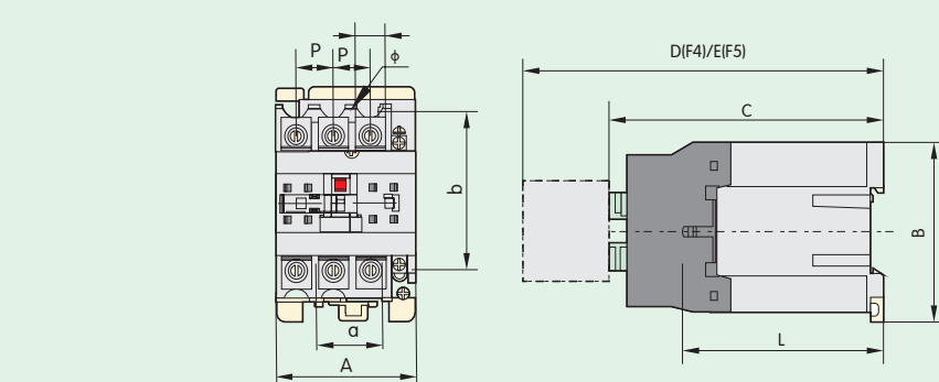
图4 NC1-40Z~95Z外形及安装尺寸
