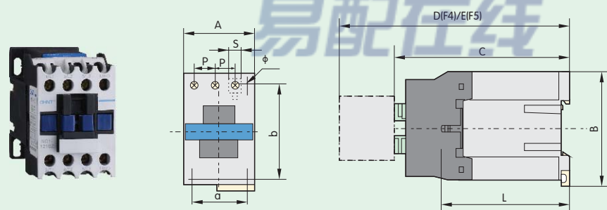
图3 NC1-09Z~32Z外形及安装尺寸
