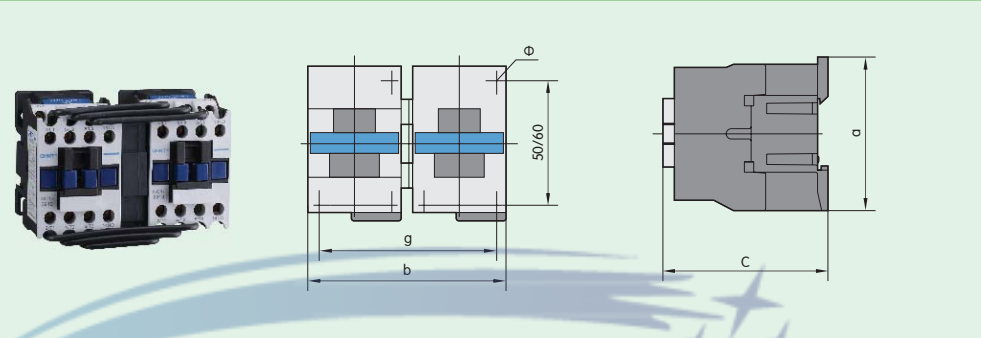
图6 NC1-40N~95N外形及安装尺寸
