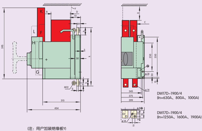
图16-2 DW17D-1900/4( I_n=630\sim 1900 )四极固定式垂直接线
