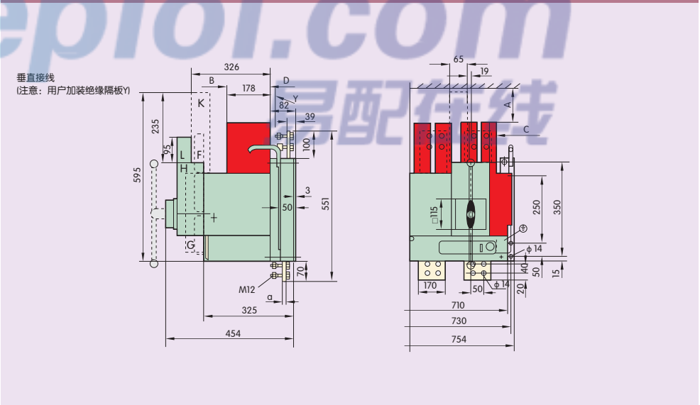
图16-4 DW17D-2900/4(In=2000A~2500A)四极固定垂直接线
