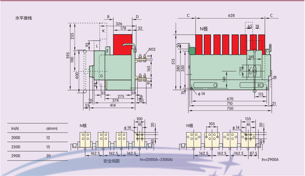
图16-3 DW17D-2900/4(In=2000A~2900A)四极固定水平接线
