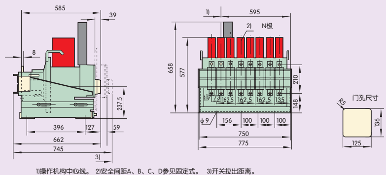
图16-7 DW17D-2900/4( I_n=2000A、2500A )四极抽屉式接线
