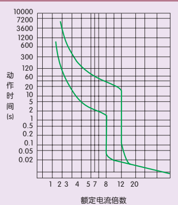
图11 NM1-1250动作特性曲线
