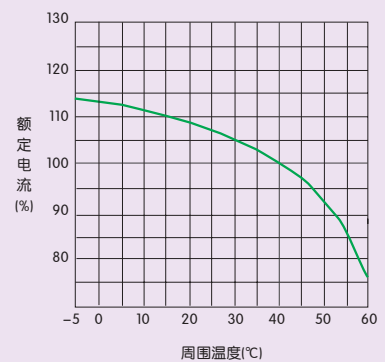
图6 NM1-250温度补偿曲线
