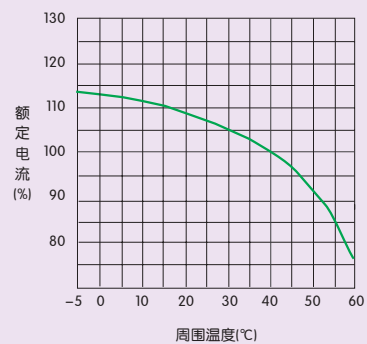
图12 NM1-1250温度补偿曲线
