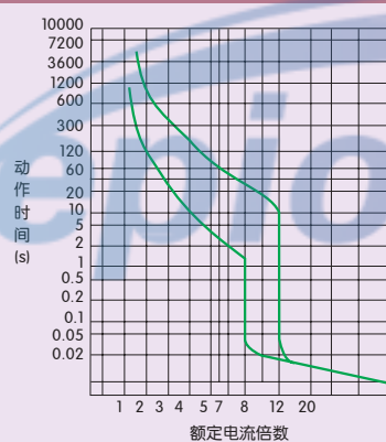
图9 NM1-630、800动作特性曲线
