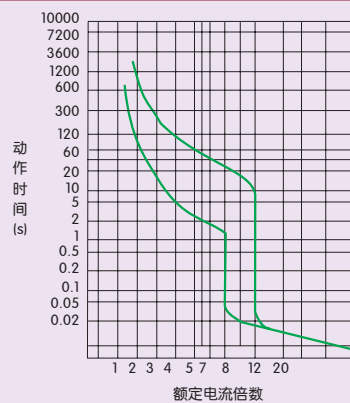
图7 NM1-400动作特性曲线
