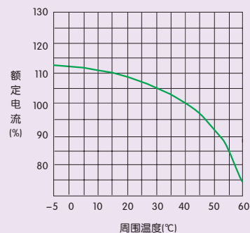
图8 NM1-400温度补偿曲线
